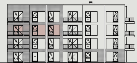
Ansicht Süd
